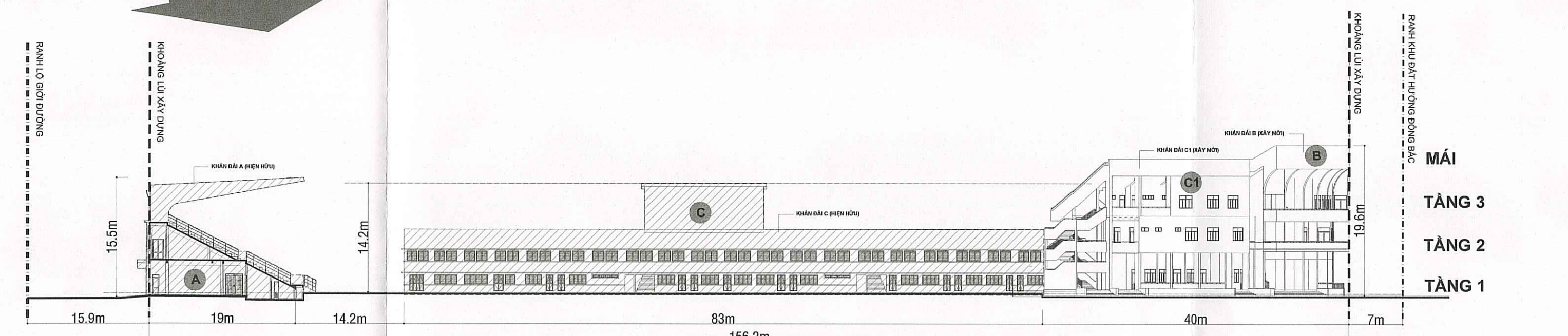
MẶT ĐỨNG TOÀN KHU NHÌN TỪ TRỰC ĐƯỜNG ĐÀO DUY TỪ - TL:1/500
