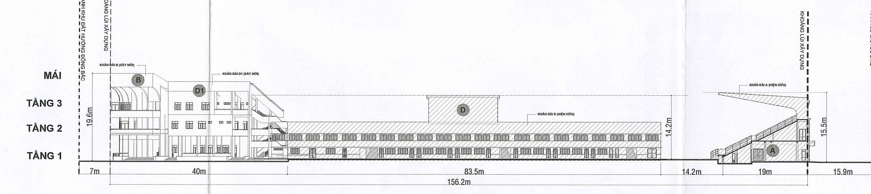
MẶT ĐỨNG TOÀN KHU NHÌN TỪ TRỰC ĐƯỜNG TÂN PHƯỚC TL: 1/500
