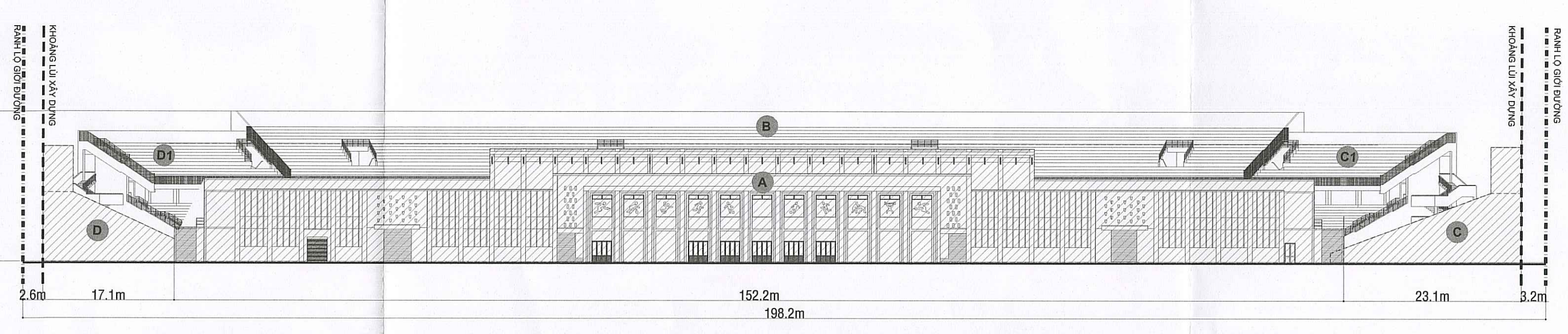
MẶT ĐỨNG TOÀN KHU NHÌN TỪ TRỰC ĐƯỜNG NGUYỄN KIM - TL: 1/500
