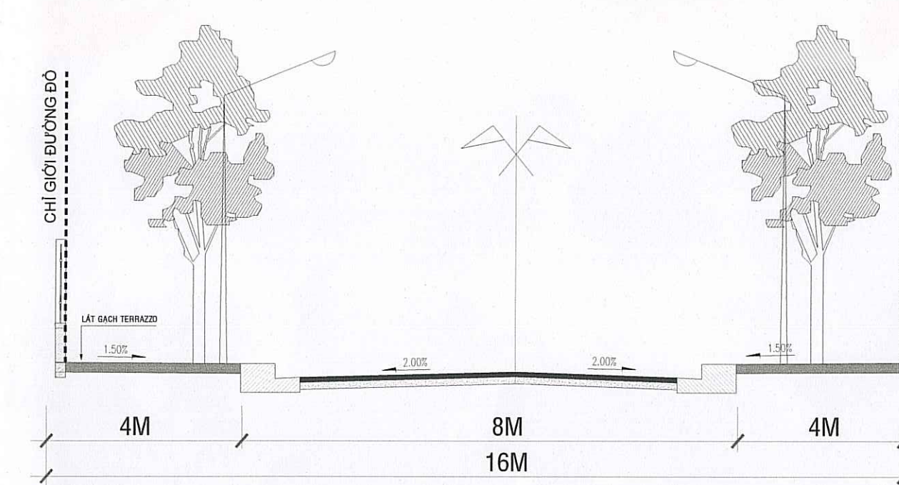
MẶT CẮT C-C - ĐƯỜNG ĐÀO DUY TỬ - TỶ LỆ 1/100
